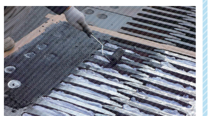
鋼製伸縮装置の省工程滑り止めコート材
