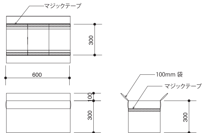
製品図面
