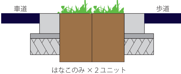
地先タイプ両面縁石抑え | HKM-040625
