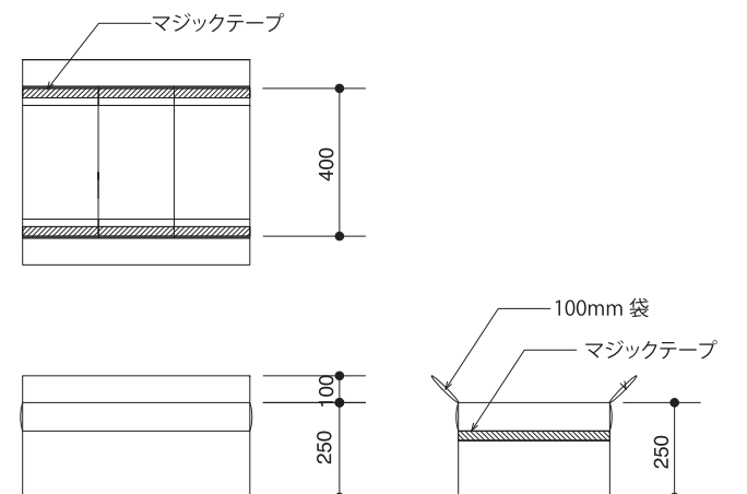
製品図面
