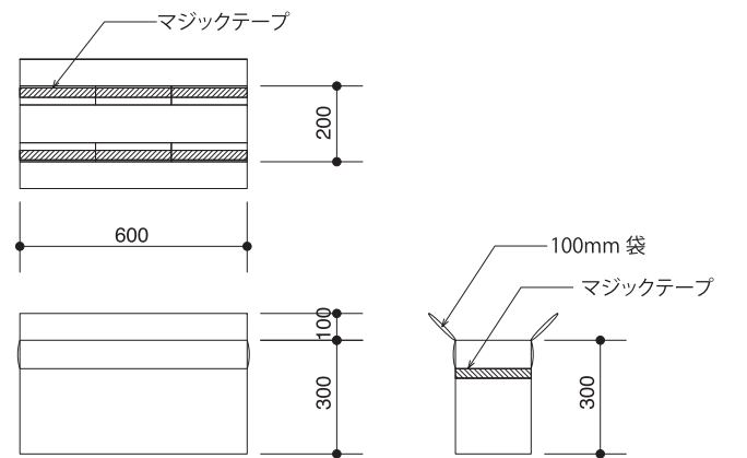
製品図面
